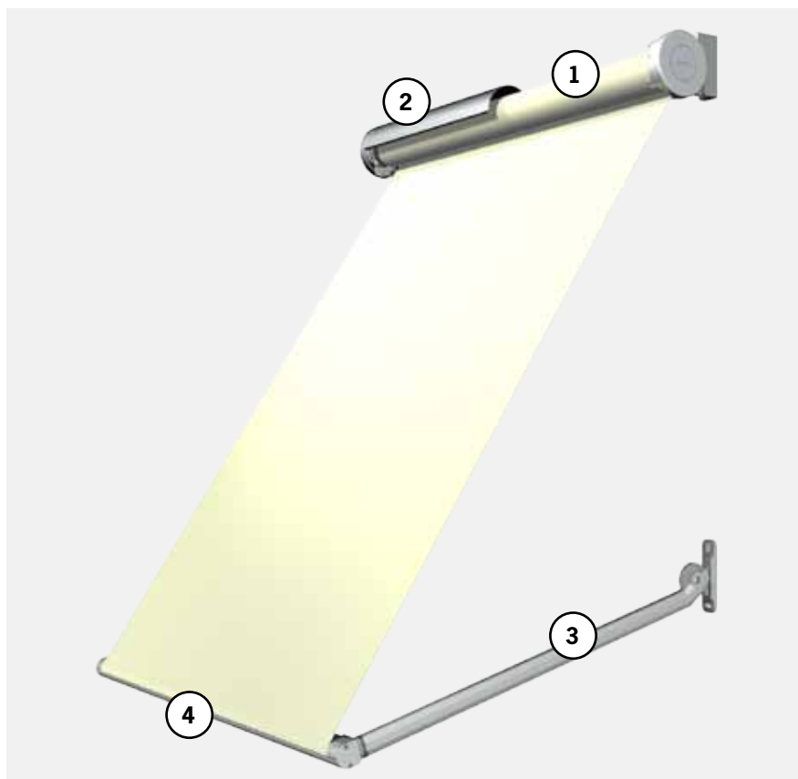
Box (Abdeckung) mit Montage nach oben
