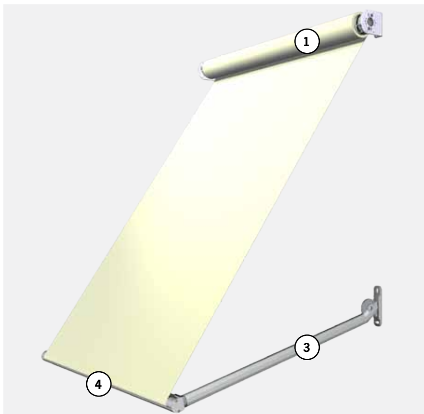
Design Lager für Montage nach hinten
