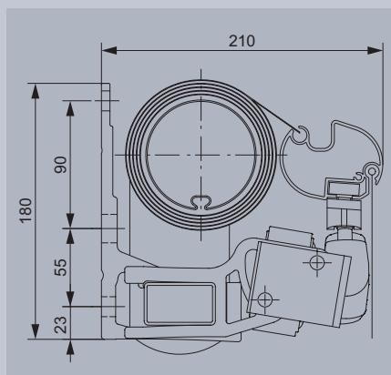
Montage mural Topas® sans toit
