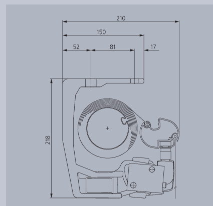
Montage au plafond Topas® sans toit
