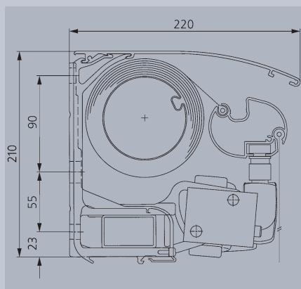
Montage mural Topas® avec toit
