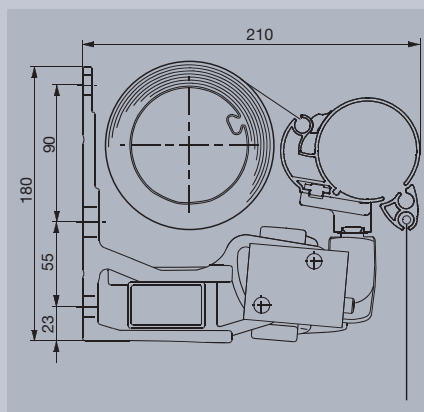
Topas® avec Volant-Plus (Option avec toit)
