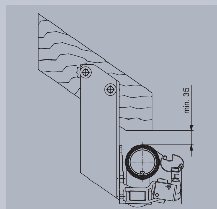
Montage sur chevrons Topas® sans toit
