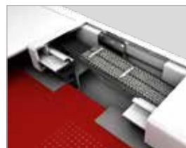
Vue de coupe - rail de guidage avec système zip et profilé en plastique à l'intérieur et courroie en tissu élastique.
